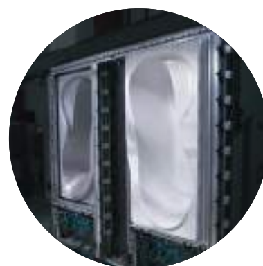
Штамповочный цех RAVAK Изготовление штампованного изделия будущей акриловой ванны с помощью технологии вертикального нагрева.
