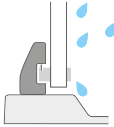
Рама в нижней части душевого угла 10°, Pivot, Blix Slim, Blix, Supernova
