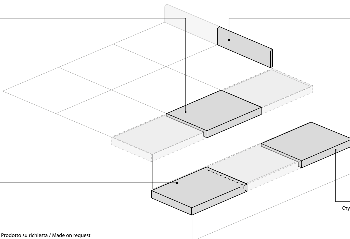
Ступень Угловая Левая ** Scalino Angolare Sx Step tread corner Sx 33x60 см ●
