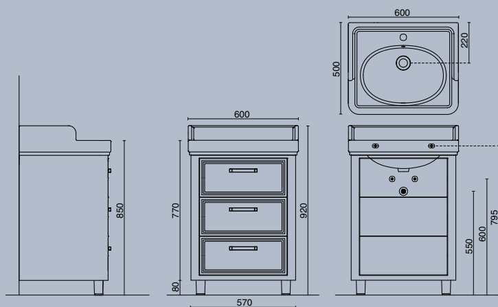
ТУМБА POMPEI ДЛЯ РАКОВИНЫ 60 CM, 3 ЯЩИКА, ЦВЕТ: БЕЛЫЙ ИЛИ ЧЕРНЫЙ ГЛЯНЕЦ
