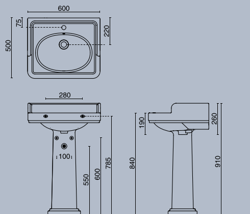
РАКОВИНА POMPEI 60 CM С ПЬЕДЕСТАЛОМ
