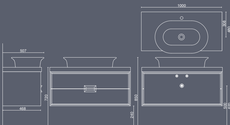
ТУМБА CANALETTO, 2 ЯЩИКА (ПОДХОДИТ ДЛЯ РАКОВИН BUONGIORNO)
