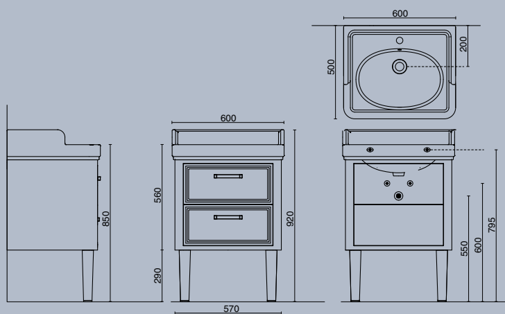
ТУМБА POMPEI ДЛЯ РАКОВИНЫ 60 CM, 2 ЯЩИКА, ЦВЕТ: БЕЛЫЙ ИЛИ ЧЕРНЫЙ ГЛЯНЕЦ
