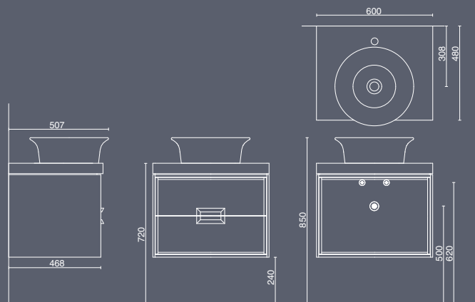
ТУМБА CANALETTO, 2 ЯЩИКА (ПОДХОДИТ ДЛЯ РАКОВИН BUONGIORNO)
