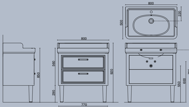
ТУМБА ДЛЯ РАКОВИНЫ 80 CM, 2 ЯЩИКА, ЦВЕТ: БЕЛЫЙ ИЛИ ЧЕРНЫЙ ГЛЯНЕЦ
