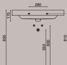
РАКОВИНА BUONGIORNO 80 CM
