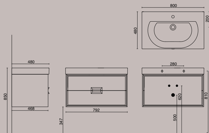
ТУМБА CANALETTO, 2 ЯЩИКА (ПОДХОДИТ ДЛЯ РАКОВИН BUONGIORNO)
