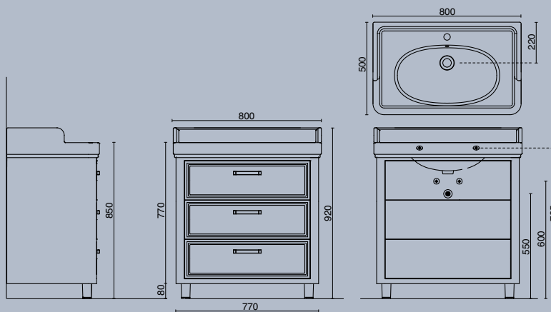
ТУМБА POMPEI ДЛЯ РАКОВИНЫ 80 CM, 3 ЯЩИКА, ЦВЕТ: БЕЛЫЙ ИЛИ ЧЕРНЫЙ ГЛЯНЕЦ
