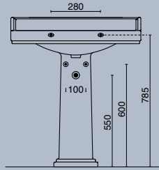
РАКОВИНА POMPEI 80 CM С ПЬЕДЕСТАЛОМ
