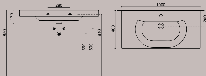
ПАКОВИНА BUONGIORNO 100 CM
