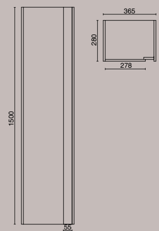
ПЕНАЛ BUONGIORNO 150 CM ЦВЕТ: БЕЛЫЙ, ДУБ
