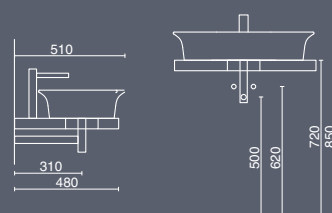
CANALETTO WASHBASIN 65X47 CM
