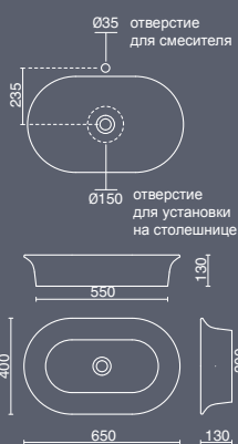
РАКОВИНА CANALETTO 65X47 CM
