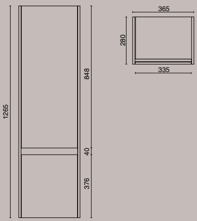
ПЕНАЛ BUONGIORNO 120 CM, 2 ДВЕРИ ЦВЕТ: БЕЛЫЙ, ДУБ
