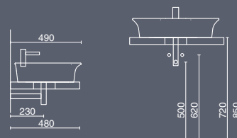
CANALETTO WASHBASIN 60X47 CM
