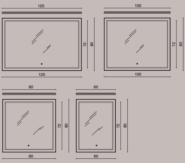
ПАНЕЛЬ С ЗЕРКАЛОМ LED 120X80 CM ПАНЕЛЬ С ЗЕРКАЛОМ LED 100X80 CM ПАНЕЛЬ С ЗЕРКАЛОМ LED 80X80 CM ПАНЕЛЬ С ЗЕРКАЛОМ LED 60X80 CM
