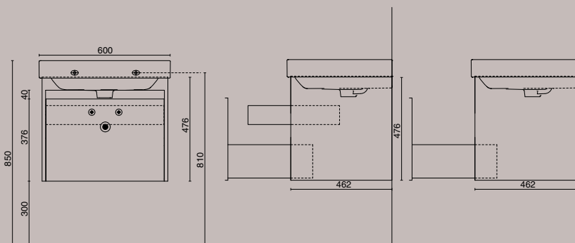
ТУМБА ПОДВЕСНАЯ BUONGIORNO 60 CM С 1 ВЫДВИЖНЫМ ЯЩИКОМ / ИЛИ + 1 ВНУТРЕННИМ ВЫДВИЖНЫМ ЯЩИКОМ, ЦВЕТ: БЕЛЫЙ, ДУБ
