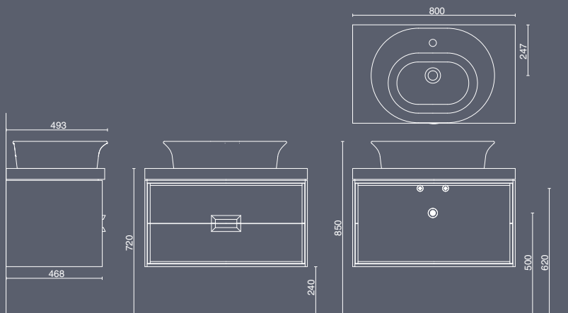
ТУМБА CANALETTO, 2 ЯЩИКА (ПОДХОДИТ ДЛЯ РАКОВИН BUONGIORNO)
