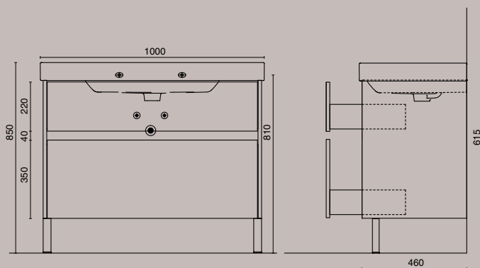
ТУМБА ПОДВЕСНАЯ BUONGIORNO 100 CM С 2 ЯЩИКАМИ, ЦВЕТ: БЕЛЫЙ, ДУБ (НОЖКИ МОЖНО ПРИОБРЕСТИ ОТДЕЛЬНО Н.200 НОЖКА ДЛЯ ТУМБЫ BUONGIORNO, 2 ЯЩИКА)
