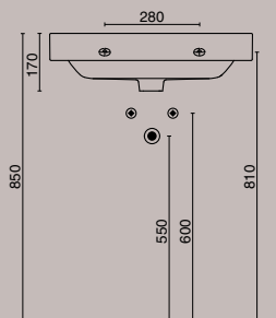
ПАКОВИНА BUONGIORNO 60 CM
