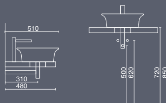
CANALETTO WASHBASIN 40X40 CM
