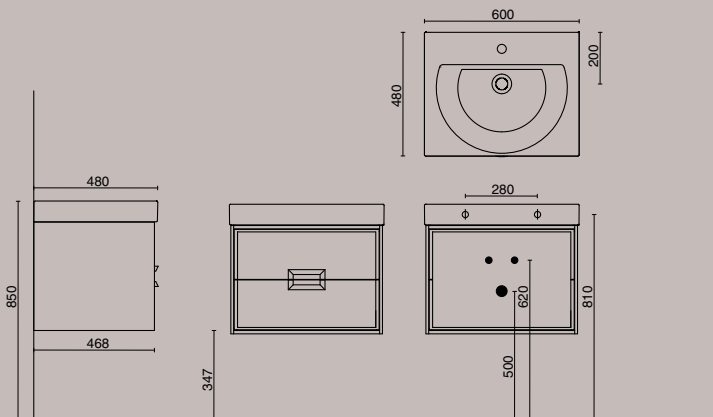
ТУМБА CANALETTO, 2 ЯЩИКА (ПОДХОДИТ ДЛЯ РАКОВИН BUONGIORNO)
