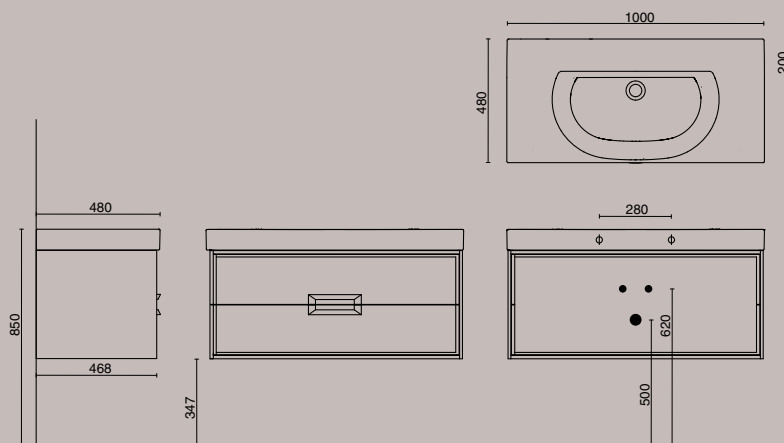
ТУМБА CANALETTO, 2 ЯЩИКА (ПОДХОДИТ ДЛЯ РАКОВИН BUONGIORNO)
